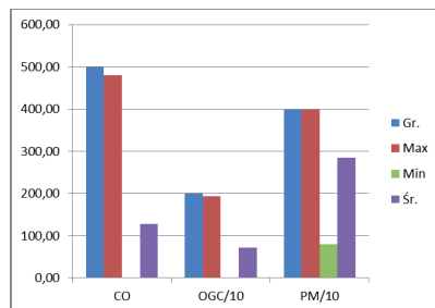
Rys. 3. Emisje tlenku węgla CO, lotnych związków organicznych OGC, pyłu całkowitego PM z kotłów węglowych automatycznie zasilanych paliwem, mg/m 3 (10% O 2 , 0°C, 1013 mbar)
