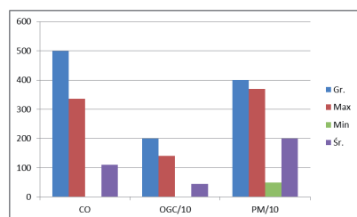
Rys. 2. Emisje tlenku węgla CO, lotnych związków organicznych OGC, pyłu całkowitego PM z kotłów automatycznie zasilanych pelletem drzewnym, mg/m 3 (10% O 2 , 0°C, 1013 mbar)
