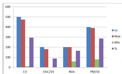
Rys. 4. Sezonowe emisje tlenku węgla CO, lotnych związków organicznych OGC, pyłu całkowitego PM z kotłów automatycznie zasilanych pelletem drzewnym, mg/m 3 (10% O 2 , 0°C, 1013 mbar)
