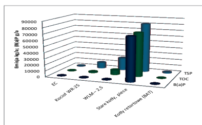
Rys. 1. Porównanie emisji z różnych instalacji węglowych, zasilającej w ciepło użytkowe przykładowe „osiedle 5 tys. mieszkańców”
