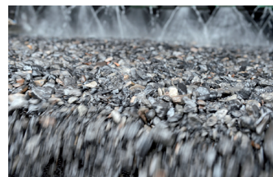
Fot. 2. Jeden z etapów procesu przetwarzania odpadów wydobywczych na instalacji zakładu Z-12 „HALDEX – Panewniki”
