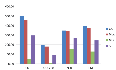
Rys. 5. Sezonowe emisje tlenku węgla CO, lotnych związków organicznych OGC, pyłu całkowitego PM z kotłów węglowych automatycznie zasilanych paliwem, mg/m 3 (10% O 2 , 0°C, 1013 mbar)
